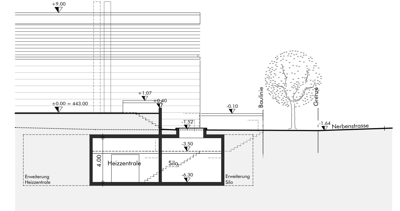
Schnitt B-B
